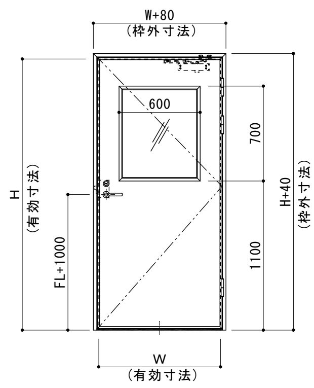
外観図
