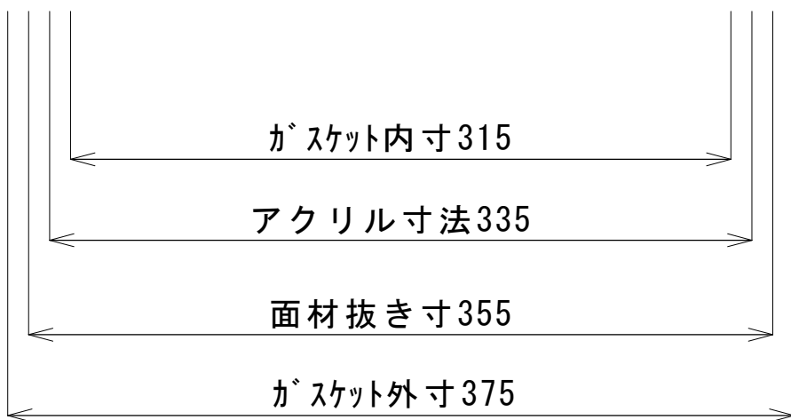
スイングドア標準窓ガasket正面詳細図
