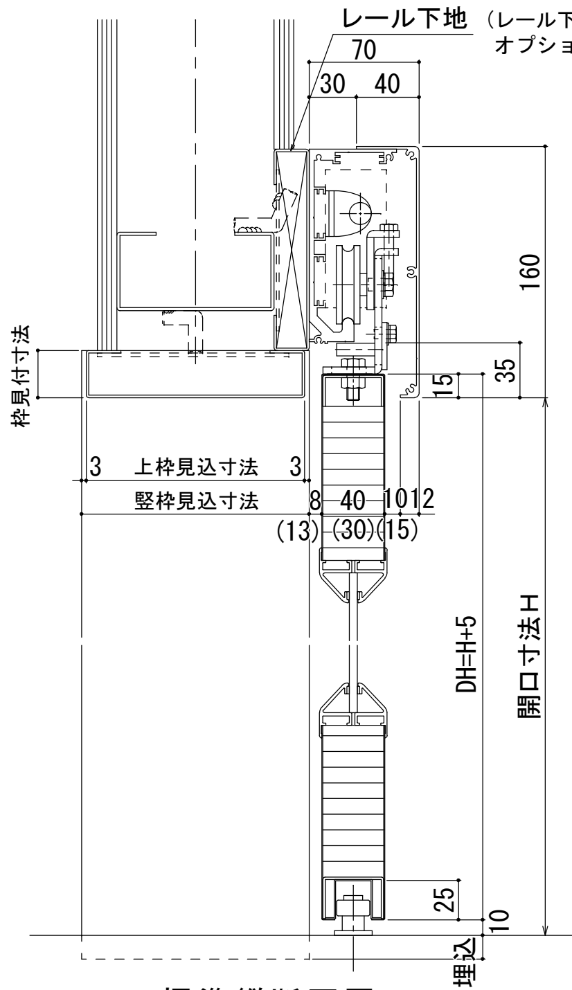
標準縦断面図
