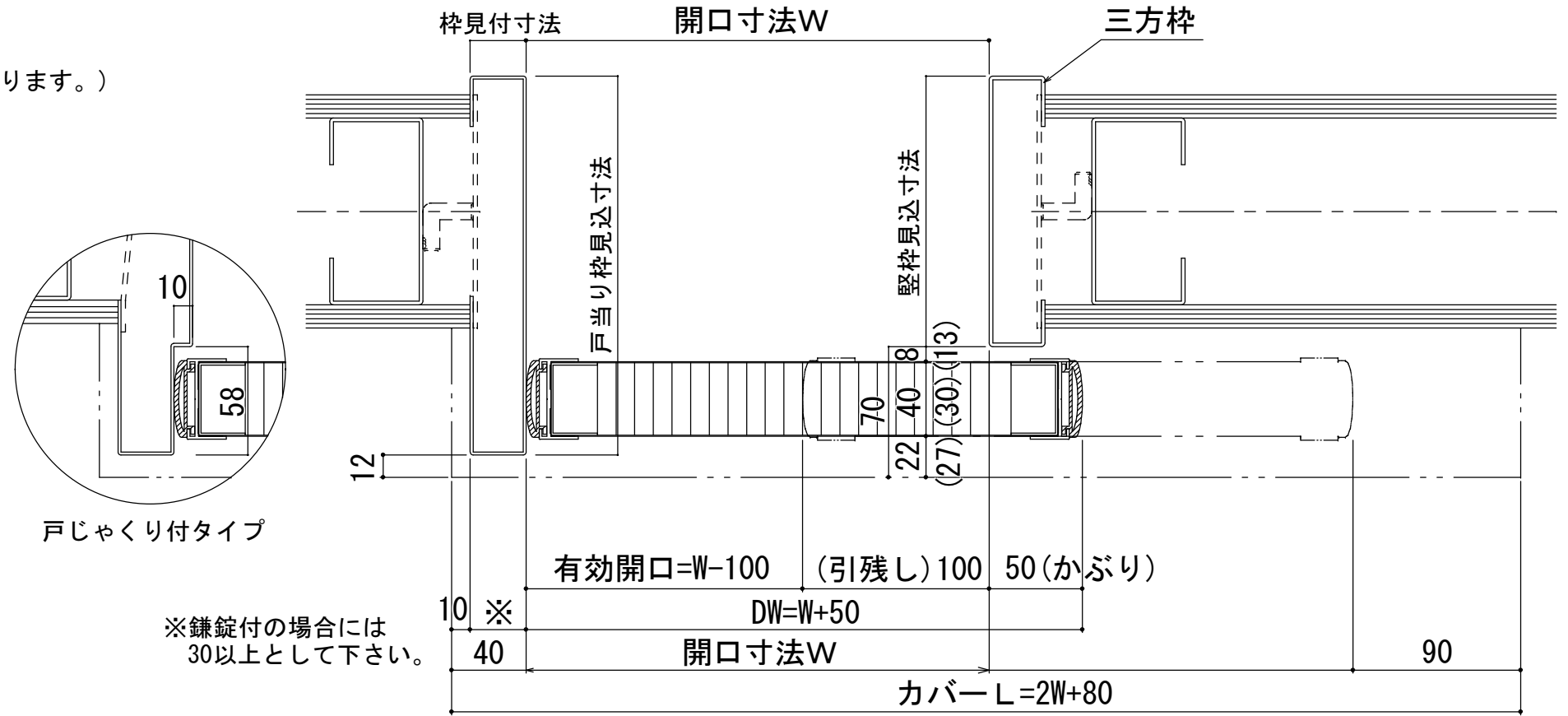
右引標準横断面図
