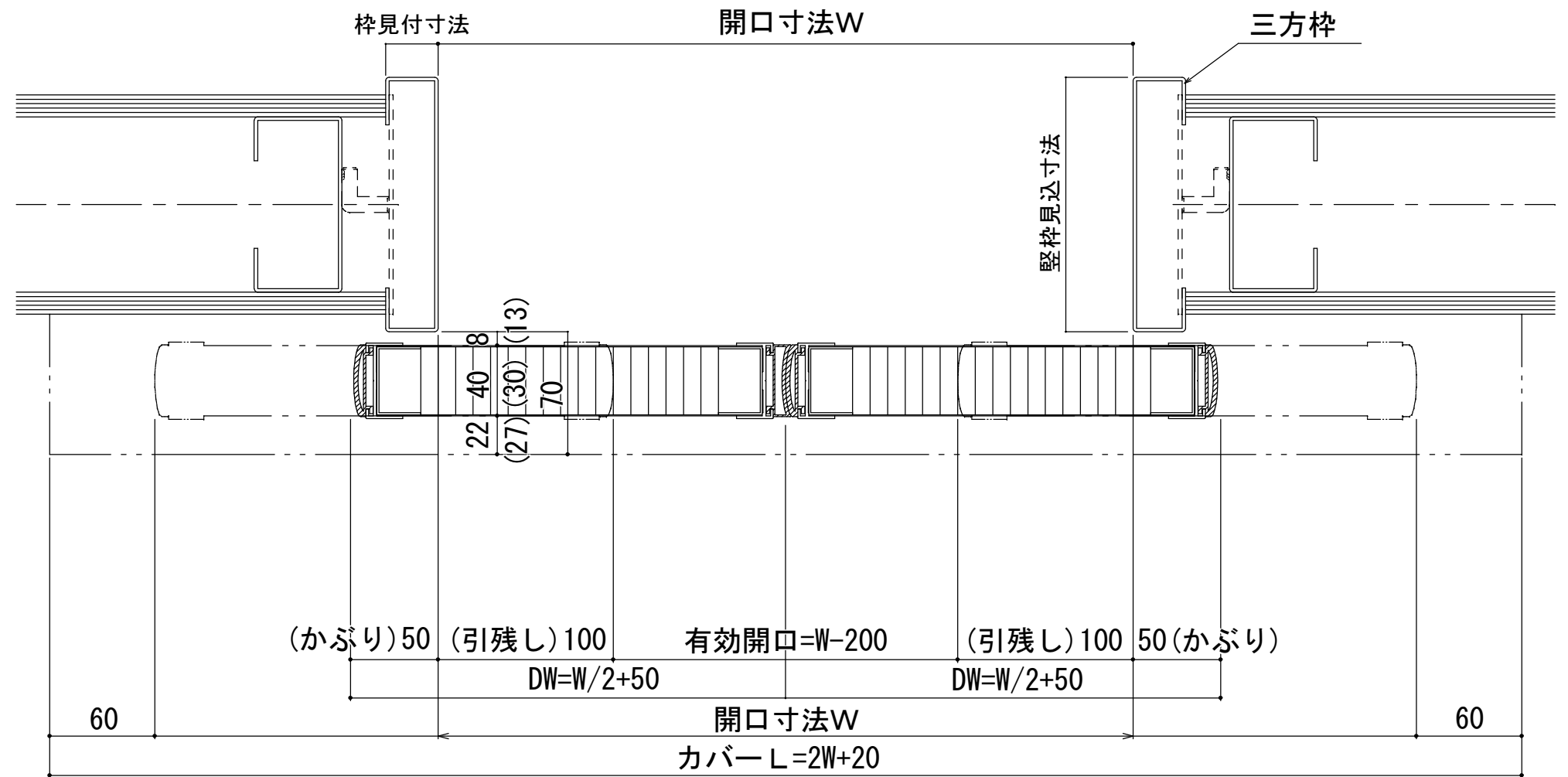
両引標準横断面図
