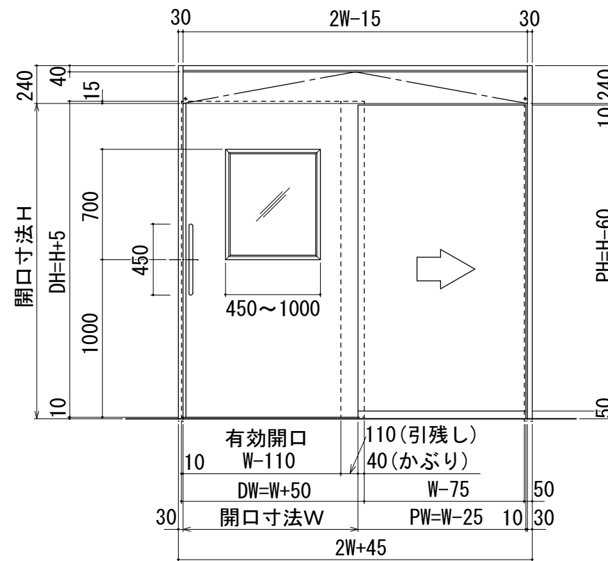
片面戸袋片面壁式右引正面図
