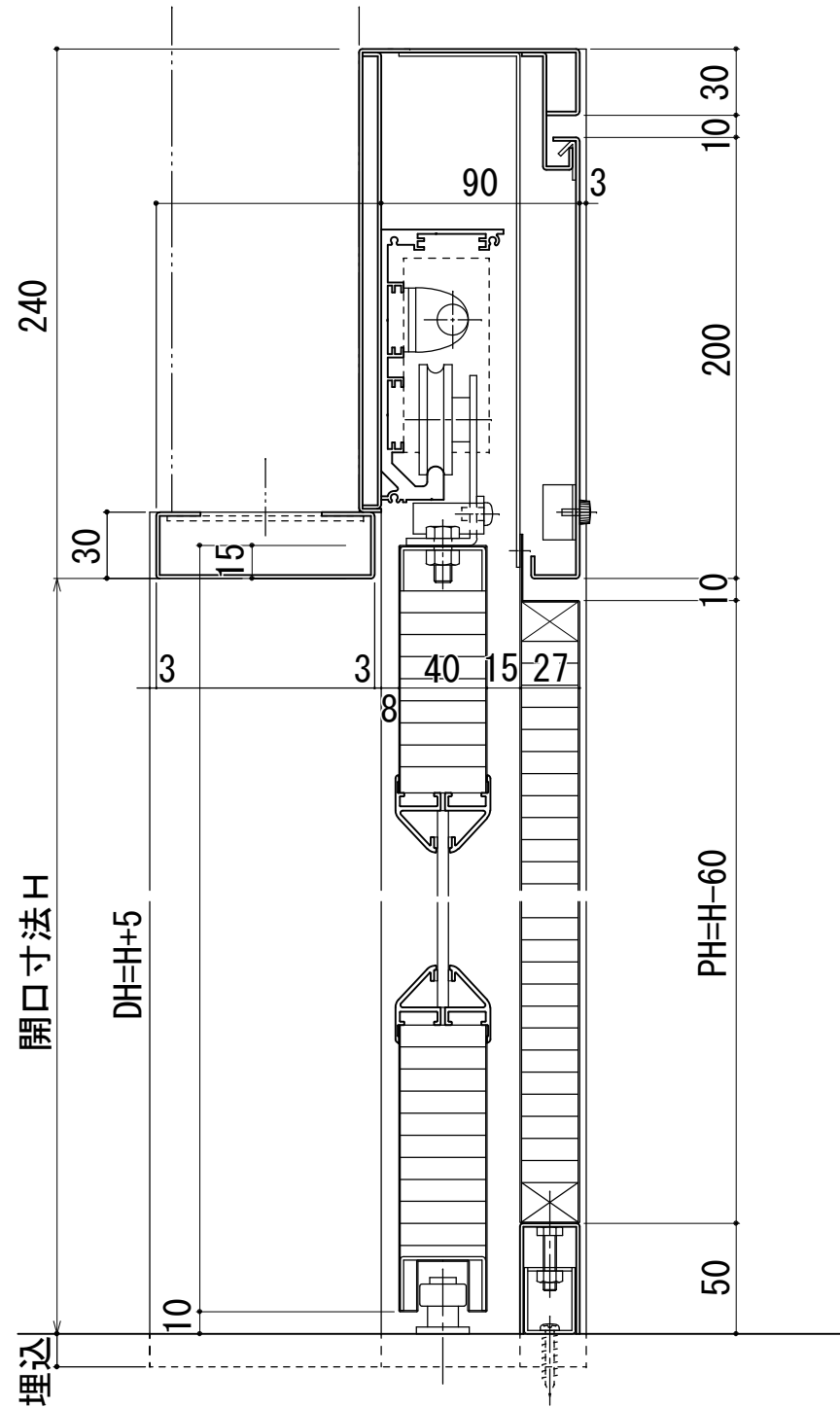
片面戸袋片面壁式縦断面図
