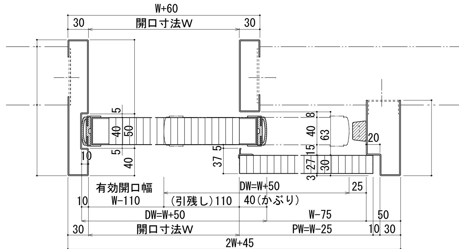
片面戸袋片面壁式右引横断面図
